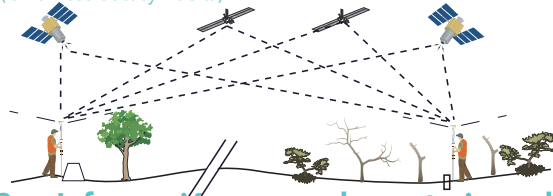
Figura 21. Nivelación diferencial con receptores GNSS. Símbolos cortesía de la integración y la red de aplicaciones ( ian.umces.edu/symbols/ ).
